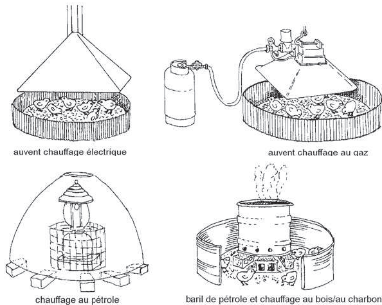
Figure 23 : Sources de chaleur possibles d'une éleveuse
